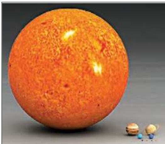
مقایسه اندازه خورشید و سیاره‌های منظومه خورشیدی
